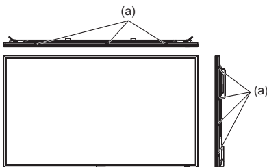
(a) ベゼルの固定するネジ (55 インチ : M3、14 個、70 インチ : M3、18 個)
