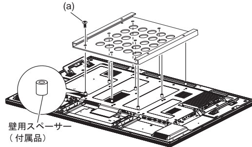
(a) 壁用スペーサーを取り付けるネジ（M6、9個）
