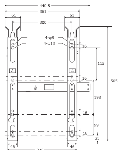
テレビ背面の金具取付ネジ部の 左右の間隔が 300mmの場合
