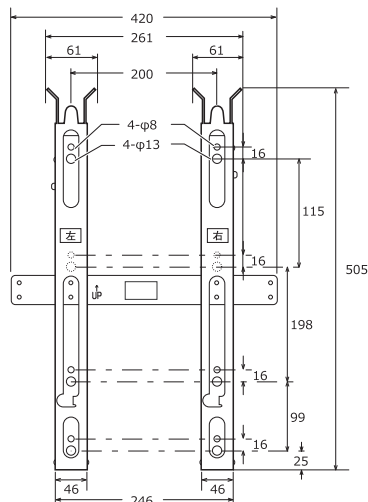
テレビ背面の金具取付ネジ部の 左右の間隔が 200mmの場合
