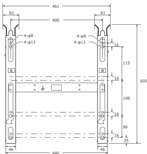
テレビ背面の金具取付ネジ部の 左右の間隔が 400mmの場合
