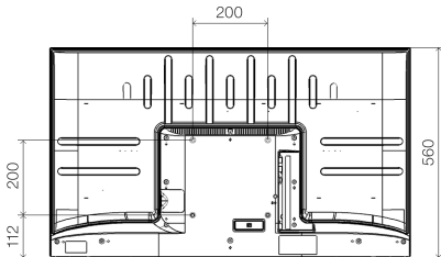
43型C350 寸法図(mm)
