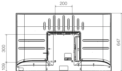
50型C350 寸法图(mm)
