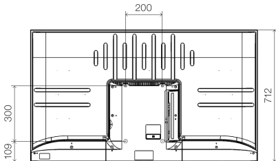
55型C350 寸法图(mm)
